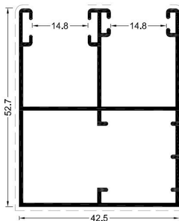
COD 9.50 G=0.74 kg/m
