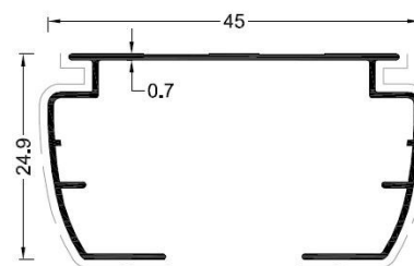
COD 5.32 G=0.24 kg/m
