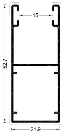
COD 9.2 G=0.44 kg/m
