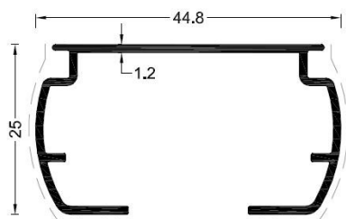
COD 5.4 G=0.35 kg/m
