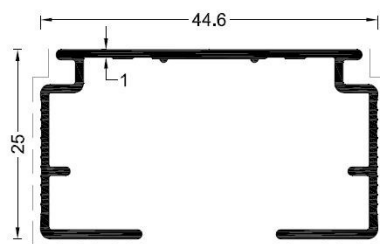
COD 5.8 G=0.35 kg/m
